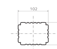
СЕЧЕНИЕ ТРУБЫ ВОДОСТОЧНОЙ 76 x 102 мм.
