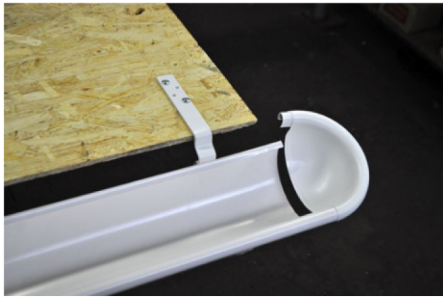
4. Сдвиньте заглушку в завитке желоба до упора..
